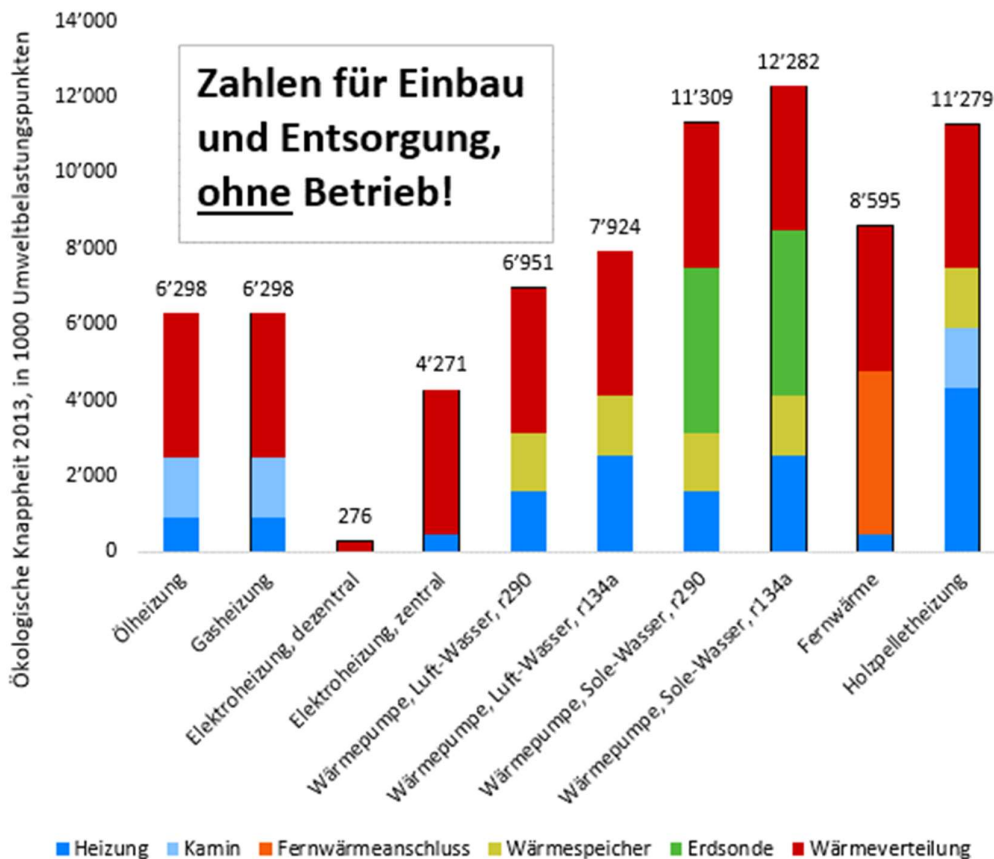
Fig. 4.13 Gesamtumweltbelastung gemäß Methode der ökologischen Knappheit 2013 auf Grund der Heizungsinstallation inklusive Entsorgung, aufgegliedert nach Bauteil und zu entsorgender Baustoffe, ohne Betrieb, in Tausend Umweltbelastungspunkten.
